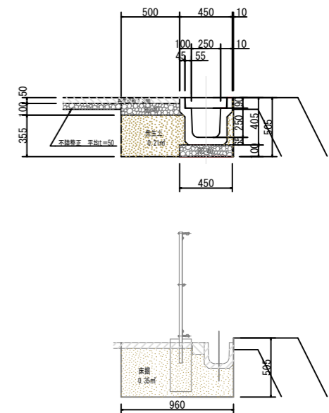
転落防止柵 単独基礎用 L=6.0m
