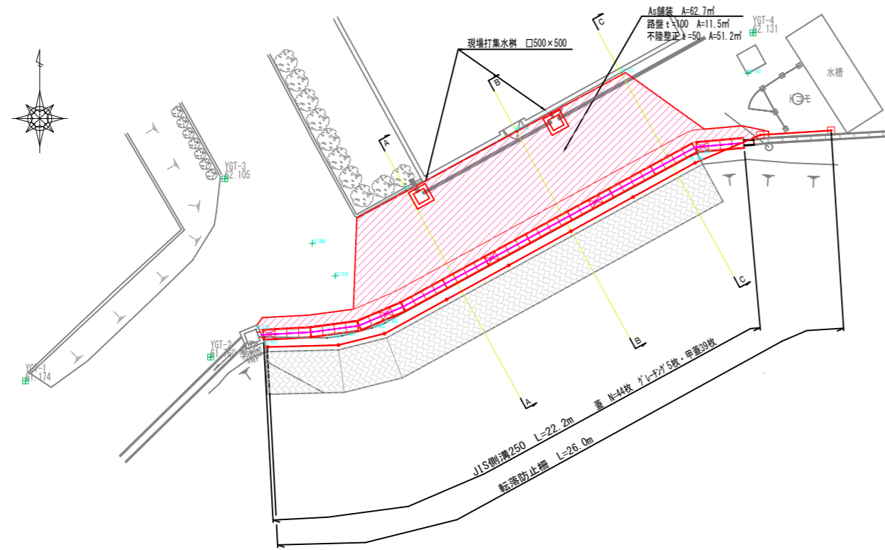
撤去平面図 S=1:100
