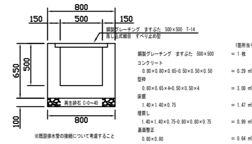
現場打集水樹 500x500
