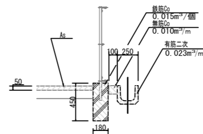
撤去構造図 S=1:20
