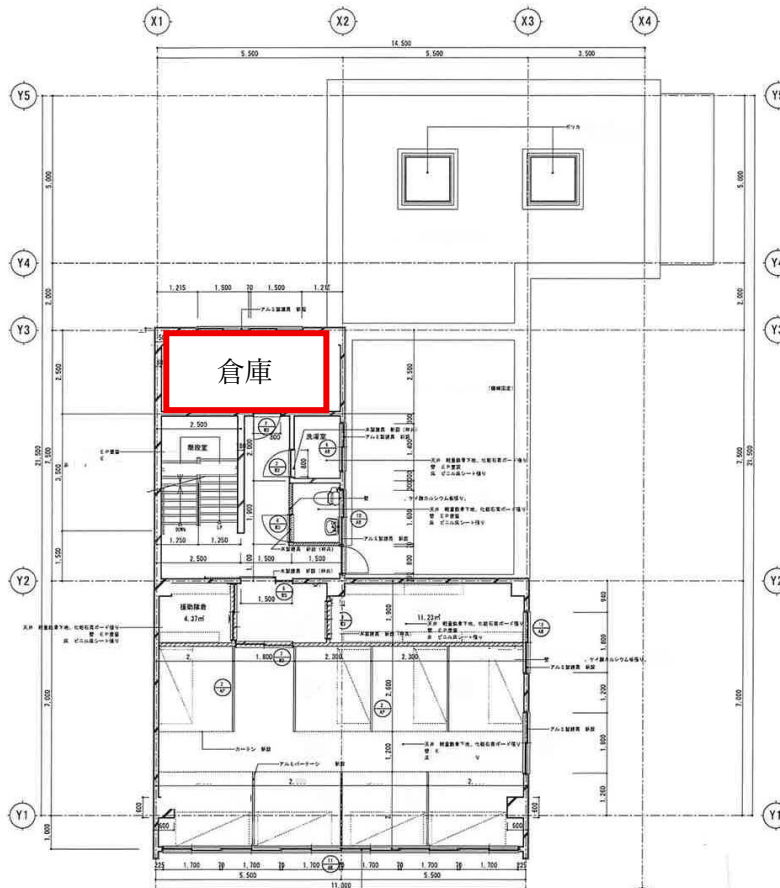
庁舎 2 階平面図
