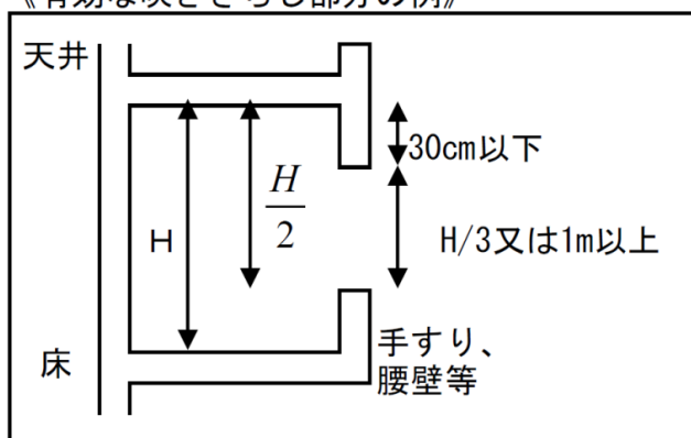
《有効な吹きさらし部分の例》
