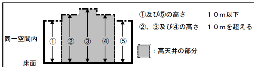
《天井までの高さの測定例》
