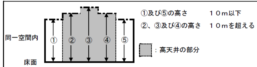
《天井までの高さの測定例》
