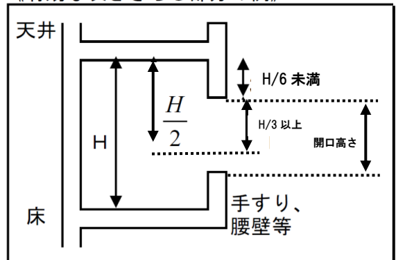
第2図 開口高さが5m以上の場合
