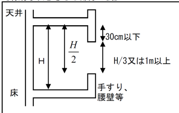
第1図 開口高さが5m未満の場合
