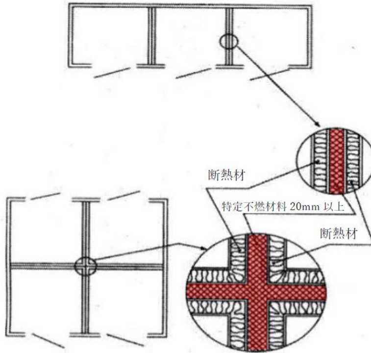
小規模サウナ室の接続
