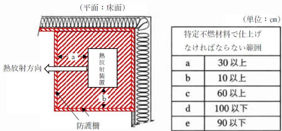
第9-2図-2 熱放射装置に面する床面の仕上げ
