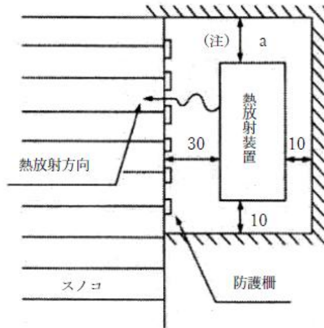
第9-4図 点検・管理空間 (単位: cm)
