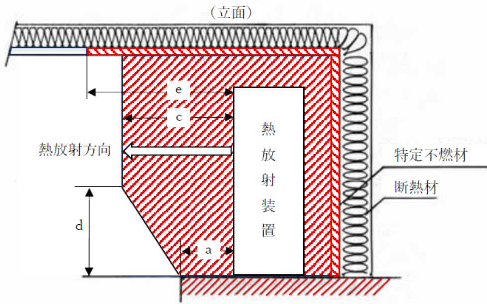
第9-2図-1 熱放射装置に面する壁面の仕上げ
