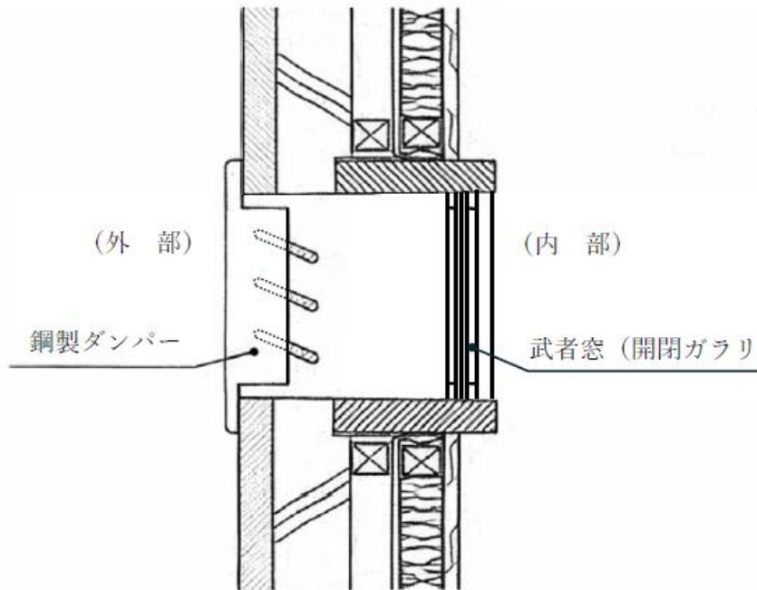
別図第 9 - 9 換気口の構造
