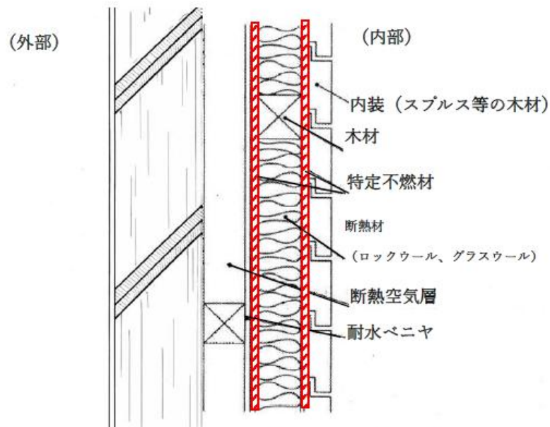
別図第9-1 対流型サウナ室及び対流型サウナ室の前室の壁体
