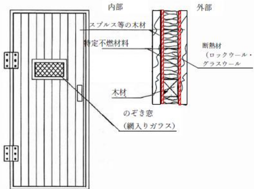
別図第9-6 対流型サウナ室の出入口とびら(その3)
