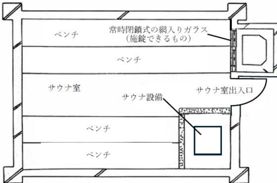
別図第 9 - 1 2 サウナ室とテレビの配置例
