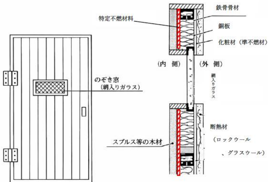
別図第9-2 対流型サウナ室の出入り口とびら (その1)
