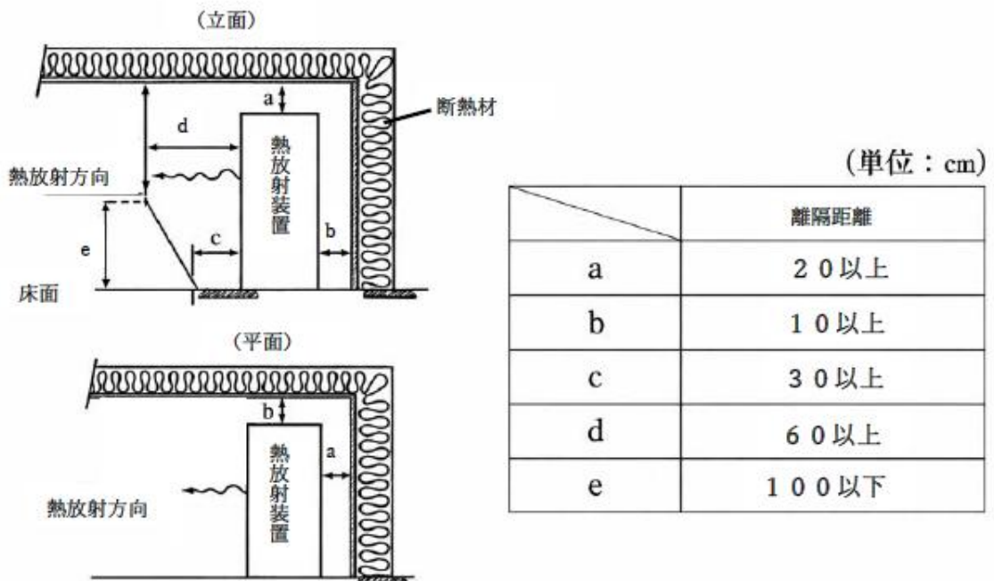
第 9 - 3 図 天井、壁面等からの離隔距離
