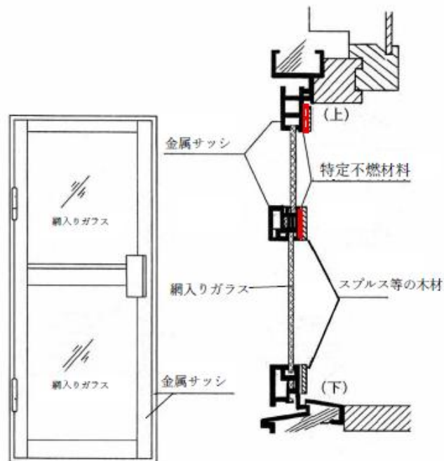
別図第9-4 対流型サウナ室の出入口とびら (その2)
