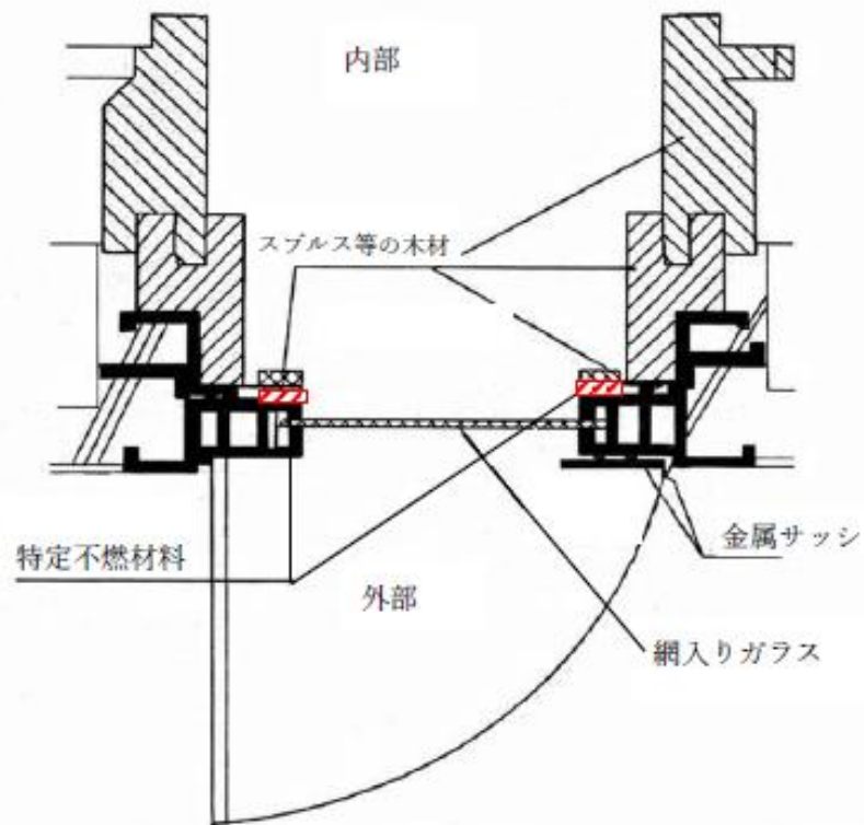
別図第9-5 対流型サウナ室の出入口のとびら(その2)取り付け方法
