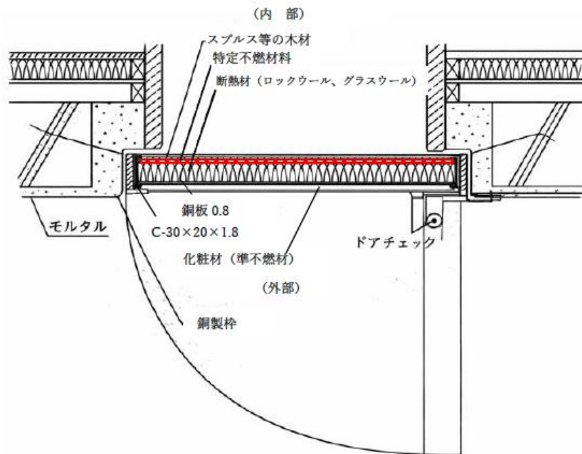
別図第9-3 対流型サウナ室の出入り口とびら (その1) 取付方法
