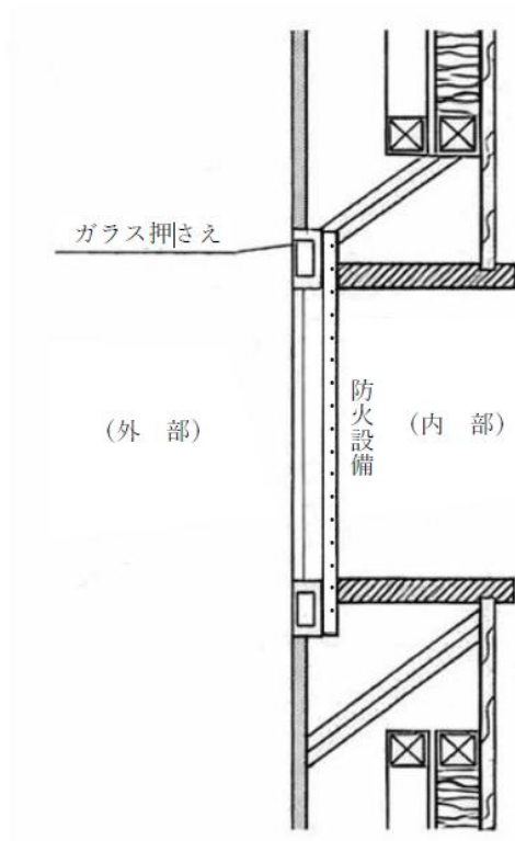
別図第9-8 洗場に面する開口部の構造
