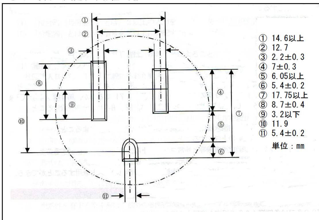
《プラグ受けの極数及び極配置の例》
